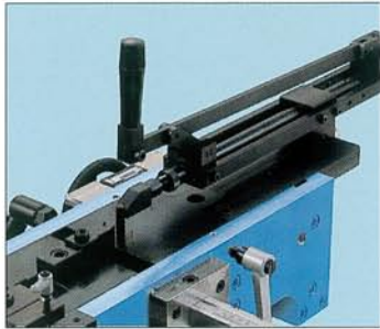
● DG-U型刃曲機にG2用曲型をセット Set up of a G2 type bending die on the Model DG-U.
