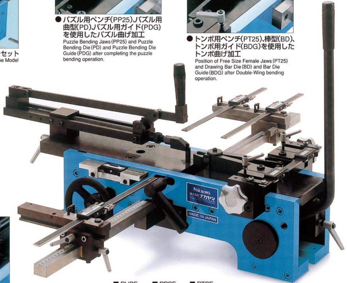
■ PU25 U字用ベンチ U-Form Bending Jaws
