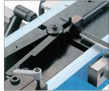
● トンボ用ベンチ(PT25)、棒型(BD)、トンボ用ガイド(BDG)を使用したトンボ曲げ加工 Position of Free Size Female Jaws (PT25) and Drawing Bar Die (BD) and Bar Die Guide (BDG) after Double-Wing bending operation.
