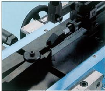
● U字用ベンチ(PU25)、絞り用曲型(UD)、長手ワンタッチ式型支え(LOTS)を使用した絞り曲げ加工 Position of U-Form Bending Jaws (PU25) and Draw Bending Die (UD) and our Long One Touch Supporter (LOTS) after bending.
