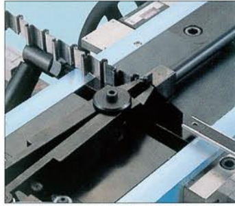
● パズル用ベンチ(PP25)、パズル用曲型(PD)、パズル用ガイド(PDG)を使用したパズル曲げ加工 Puzzle Bending Jaws (PP25) and Puzzle Bending Die (PD) and Puzzle Bending Die Guide (PDG) after completing the puzzle bending operation.
