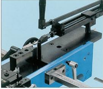
● DG-U型刃曲機にDG用曲型をセット Set up of a DG type bending die on the Model DG-U.
