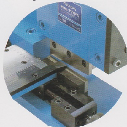
高さ30mmの刃材切断の場合 The cutting position for 30mm height steel rule.
