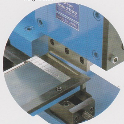
高さ100mmの刃材切断の場合 The cutting position for 100mm height steel rule.
